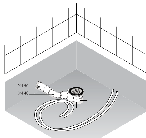
Bild 2: Beispiel für flexiblen Anschluss (Kunststoffrohr)
