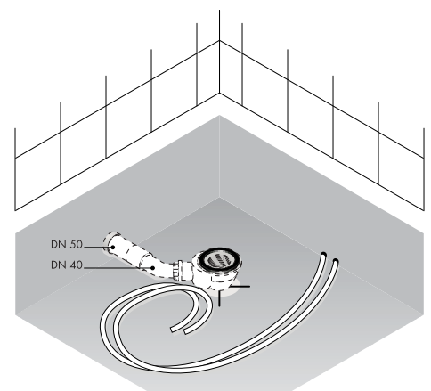
Bild 2: Beispiel für flexiblen Anschluss (Kunststoffrohr)
