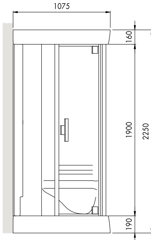
Vorderansicht
