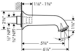
Talis C 14148XX1
