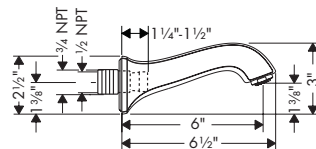
Metris C 13413XX1
