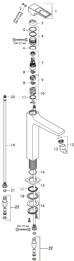
製品分解図
