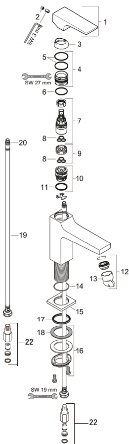
製品分解図
