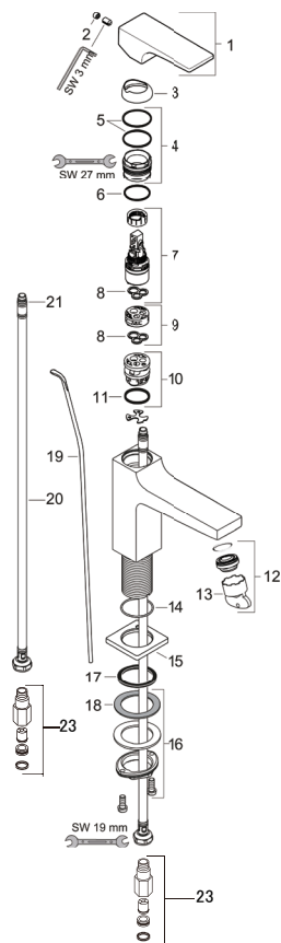
製品分解図
