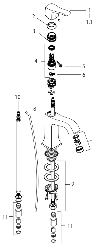
部品リスト
