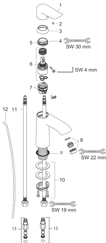
部品リスト
