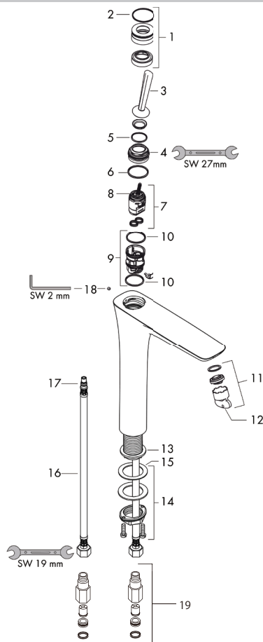
製品分解図
