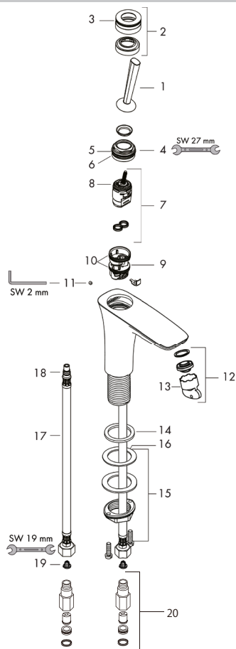
製品分解図
