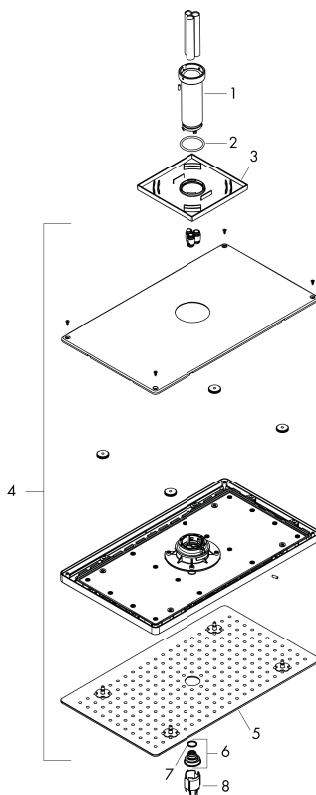
製品分解図
