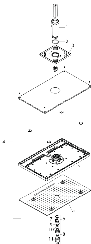
製品分解図
