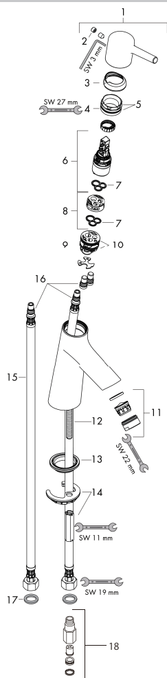
製品分解図
