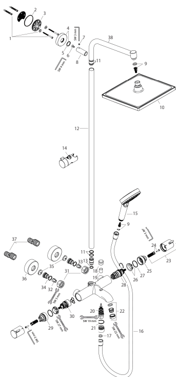
製品分解図
