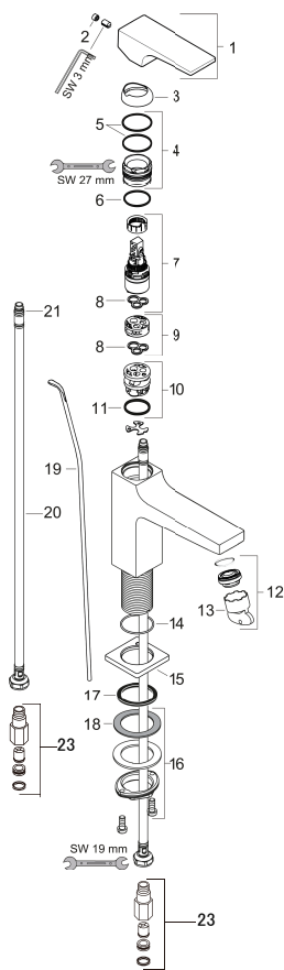
製品分解図
