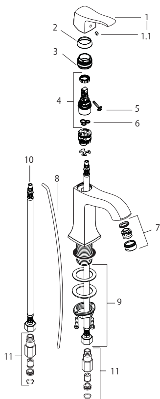
製品分解図
