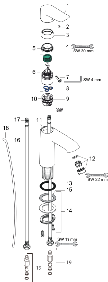
製品分解図
