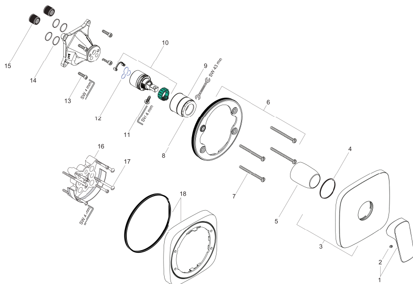
製品分解図
