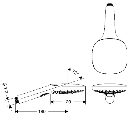
完成図
