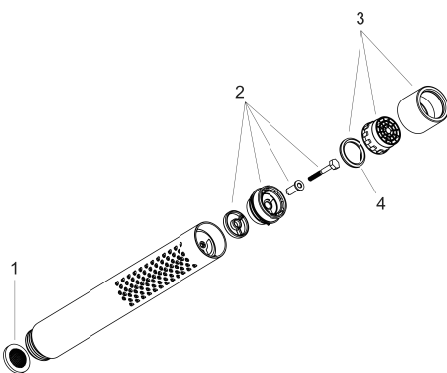
部品リスト
