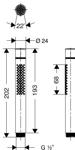
完成図
