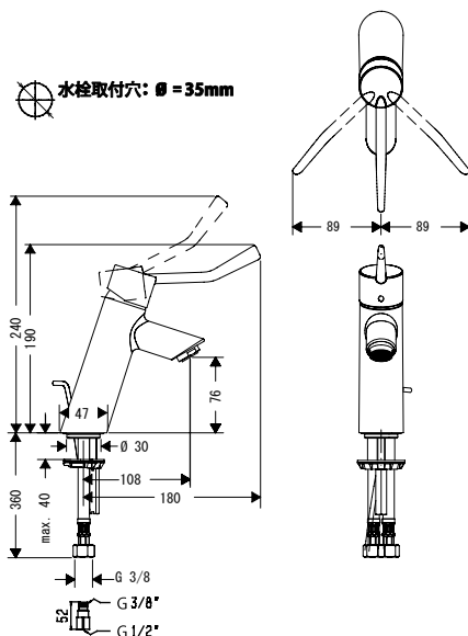
完成図
