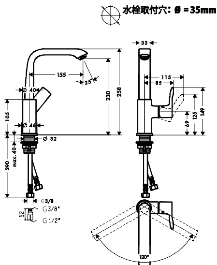
完成図
