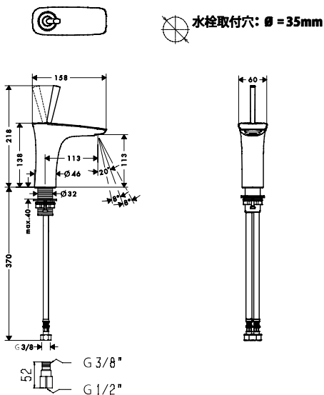
完成図
