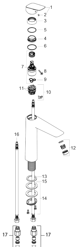
部品リスト
