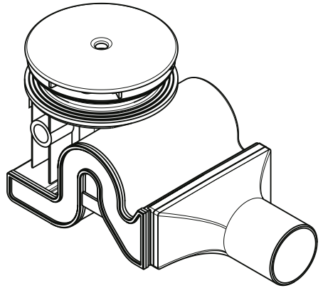
Rain Drain 60067000
