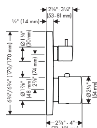
AXOR Citterio M 34725XX1
