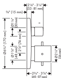
AXOR Citterio 39720XX1
