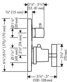
AXOR Montreux 16821XX1
