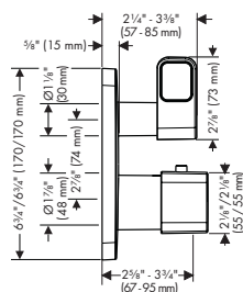
AXOR Citterio M 34725XX1
