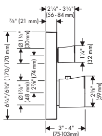
AXOR Citterio 39725XX1
