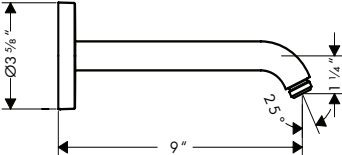
AXOR 230 Showerarm 26435XX1
