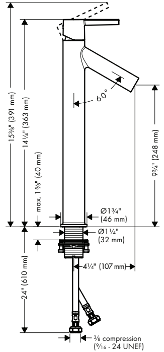
AXOR Starck 10103XX1
