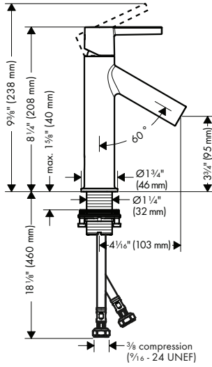
AXOR Starck 10003XX1
