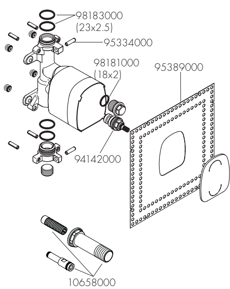
AXOR Handshower Module 10650181
