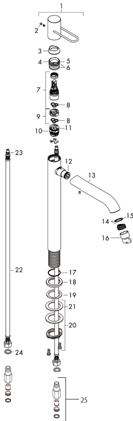
製品分解図
