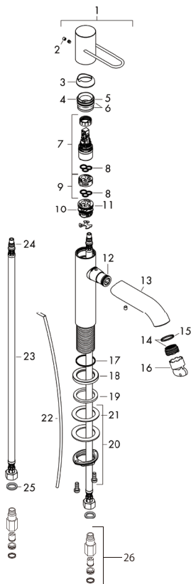
製品分解図
