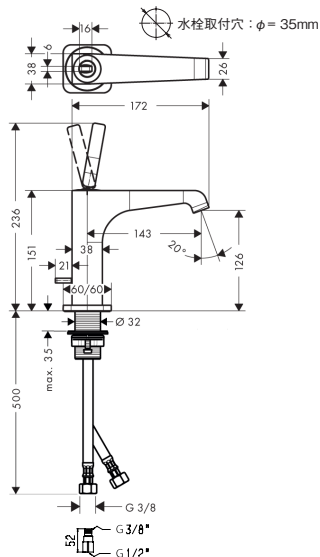
完成図
