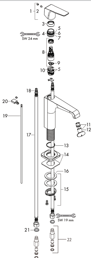
製品分解図
