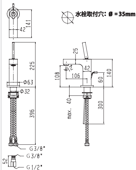
完成図
