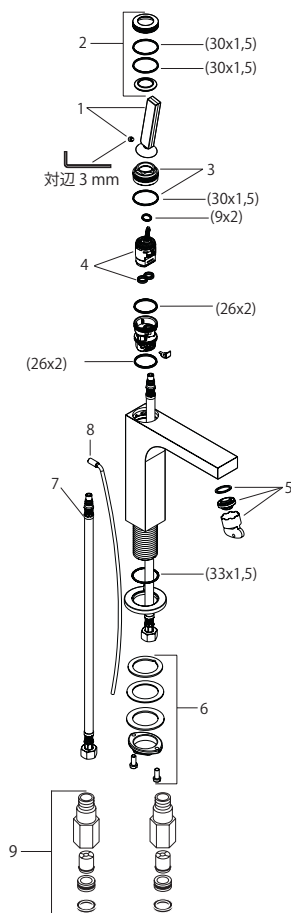
部品リスト
