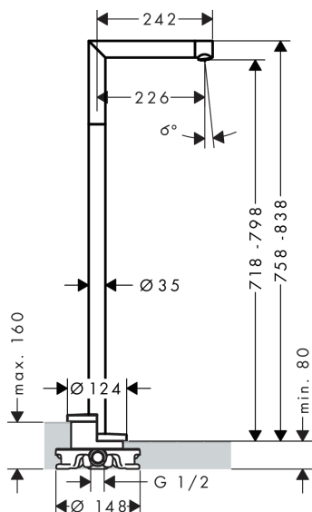
完成図
