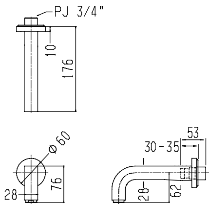
完成図
