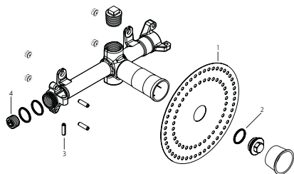
部品リスト
