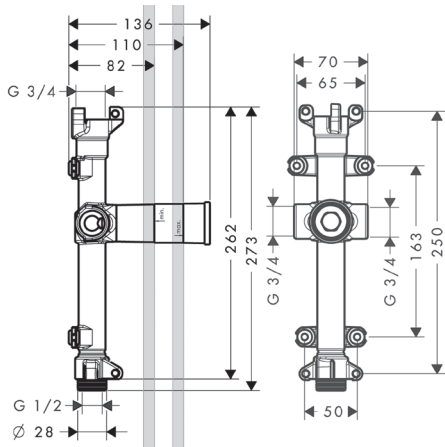
完成図
