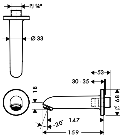
完成図
