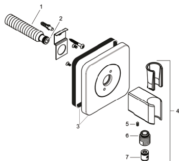
部品リスト
