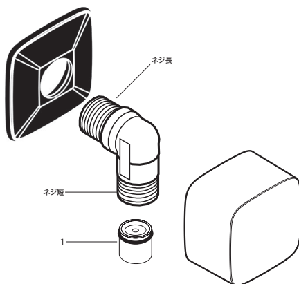
製品分解図
