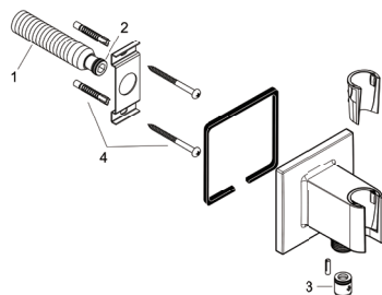
製品分解図
