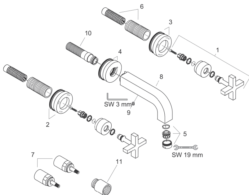
製品分解図
