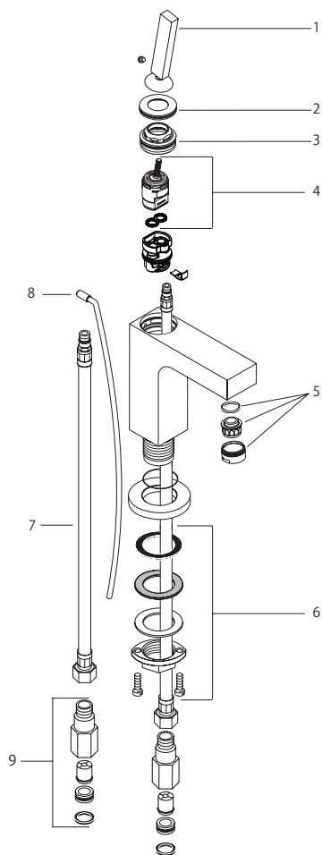
製品分解図
