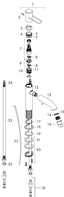
製品分解図
