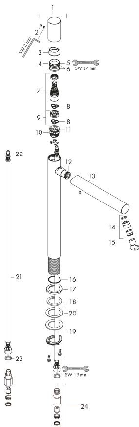
製品分解図
