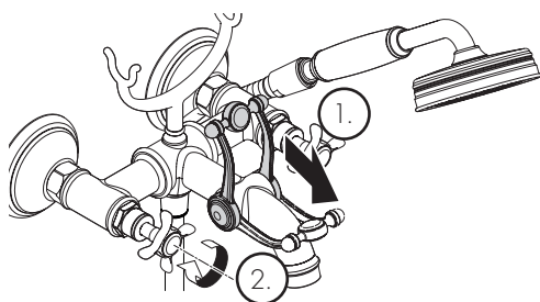
close / schließen
