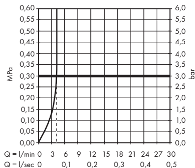
AXOR MyEdition 70 47050XXX / 47052XXX AXOR MyEdition 110 47070XXX / 47072XXX
