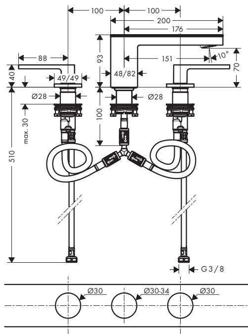
AXOR MyEdition 70 47050XXX / 47052XXX
