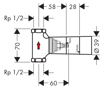
AXOR DN15 (1/2") 16974180 / 16974187
