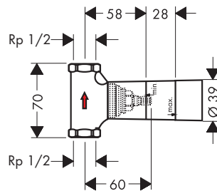
AXOR DN15 (1/2") 16973180
