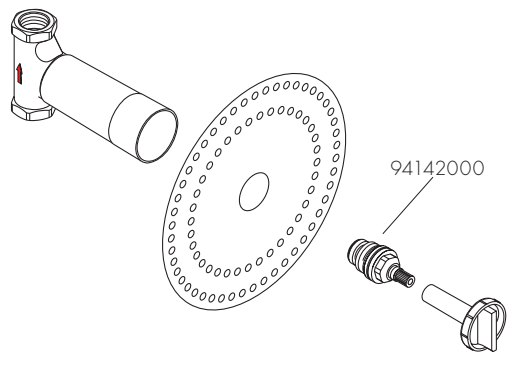
AXOR DN15 (1/2") 16973180
