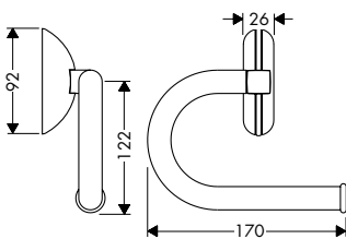
Arco 40636XXX
