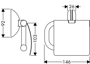
Arco 40638XXX
