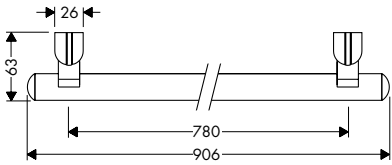
Arco 40608XXX
