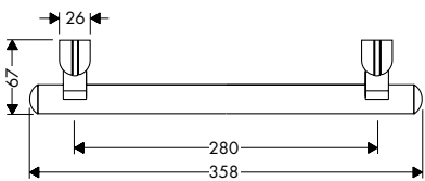
Arco 40630XXX
