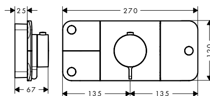
Thermostatmodul Unterputz für 3 Verbraucher
