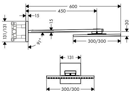
Kopfbrause 300/300 2jet mit Brausearm
