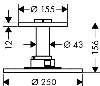
Kopfbrause 250 2jet mit Deckenanschluss
