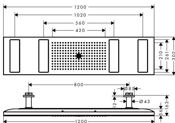
ShowerHeaven 1200/300 4jet mit Beleuchtung 2700 K
