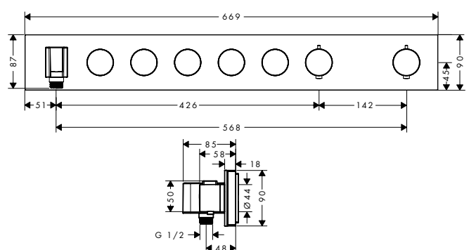
Thermostatmodul Select 670/90 Unterputz für 5 Verbraucher
