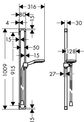
Brauseset 0,90 m mit Handbrause 120 3jet
