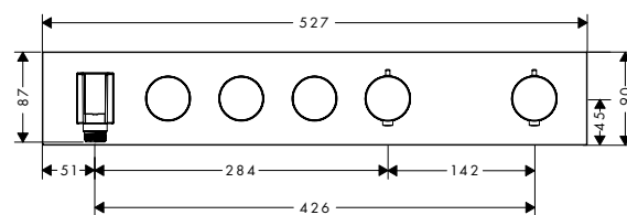
Thermostatmodul Select 530/90 Unterputz für 3 Verbraucher
