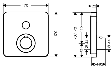
Thermostat Unterputz softcube 1 Verbraucher
