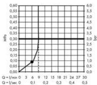
Główka prysznicowa 75 1jet EcoSmart
