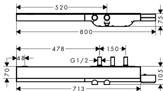
Bateria termostyczna 800, montaż natynkowo/podtynkowy
