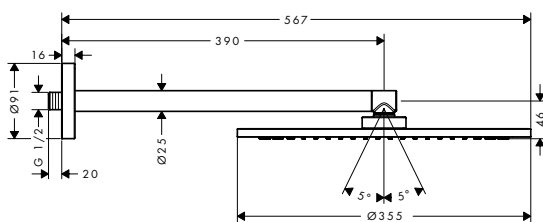
Głowica prysznicowa 350 ljet z ramieniem prysznicowym
