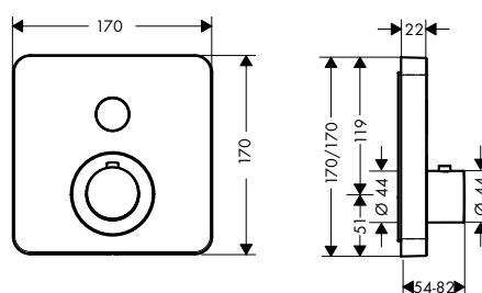
Bateria termostyczna ShowerSelect do jednego odbiornika, montaż podtynkowy
