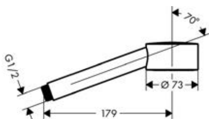
Główka prysznicowa 75 1jet EcoSmart
