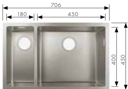
S719-U655 Onderbouw spoelbak diepte 190 mm, voor inbouwkast 800 mm # 43429,-800 Handmatige afvoergarnituur # 43924,-000 Automatische afvoergarnituur # 43934,-000
