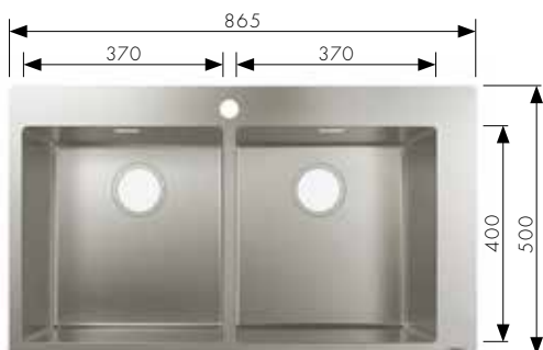
S711-F765 Inbouw spoelbak diepte 190 mm, voor inbouwkast 900 mm # 43303,-800 met één kraangang Handmatige afvoergarnituur # 43922,-000
