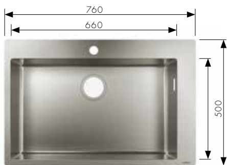
S711-F660 Inbouw spoelbak diepte 190 mm, voor inbouwkast 800 mm # 43302,-800 met één kraangang Handmatige afvoergarnituur # 43921,-000
