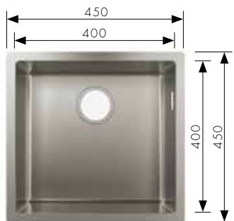
S719-U400 Onderbouw spoelbak diepte 190 mm, voor inbouwkast 500 mm # 43425,-800 Handmatige afvoergarnituur # 43925,-000 Automatische afvoergarnituur # 43935,-000
