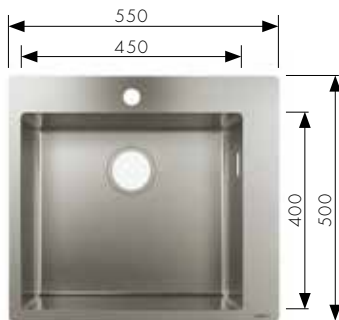
S711-F450 Inbouw spoelbak diepte 190 mm, voor inbouwkast 600 mm # 43301,-800 met één kraangat Handmatige afvoergarnituur # 43920,-000
