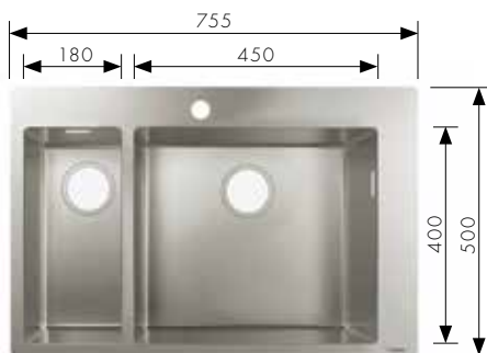
S711-F655 Inbouw spoelbak diepte 190 mm, voor inbouwkast 800 mm # 43309,-800 met één kraangang Handmatige afvoergarnituur # 43924,-000
