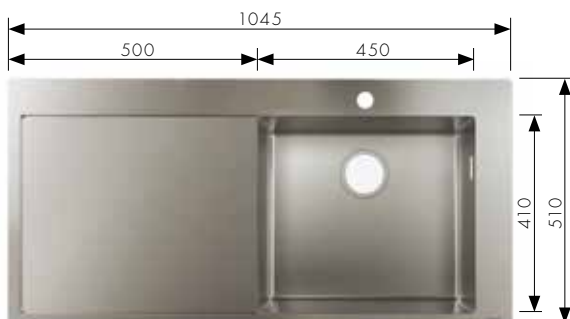
S715-F450 Inbouw spoelbak met afdruiplak diepte 190 mm, voor inbouwkast 600 mm # 43306,-800 met één kraangat Handmatige afvoergarnituur # 43920,-000
