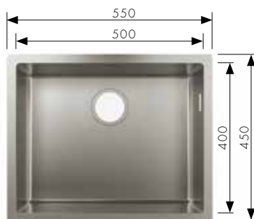
S719-U500 Onderbouw spoelbak diepte 190 mm, voor inbouwkast 600 mm # 43427,-800 Handmatige afvoergarnituur # 43926,-000 Automatische afvoergarnituur # 43936,-000
