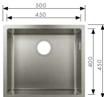
S719-U450 Onderbouw spoelbak diepte 190 mm, voor inbouwkast 600 mm # 43426,-800 Handmatige afvoergarnituur # 43920,-000 Automatische afvoergarnituur # 43930,-000
