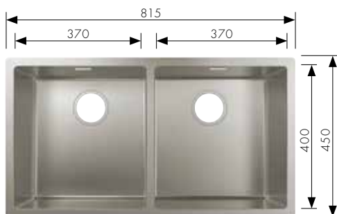
S719-U765 Onderbouw spoelbak diepte 190 mm, voor inbouwkast 900 mm # 43430,-800 Handmatige afvoergarnituur # 43922,-000 Automatische afvoergarnituur # 43932,-000
