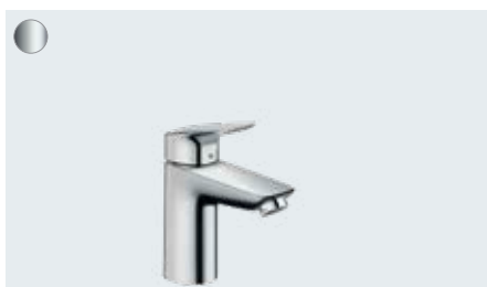
Logis ééngreeps wastafelmengkraan 100 met trekwaste # 71100, -000 ééngreeps wastafelmengkraan 100 met Push-Open afvoer # 71107, -000 ééngreeps wastafelmengkraan 100 CoolStart met trekwaste (zonder afb.) # 71102, -000 ééngreeps wastafelmengkraan 100 CoolStart zonder afvoer (zonder afb.) # 71103, -000 ééngreeps wastafelmengkraan 100 zonder afvoer # 71101, -000
