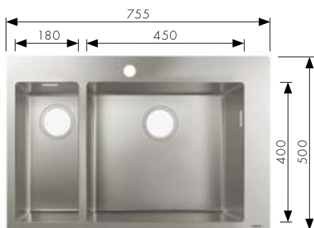
S711-F655 Inbouw en vlakkbouw spoeltafel diepte 190 mm, voor inbouwkast: 800 mm # 43309, -800, met een kraangat # 43924000 Manuele lediging
