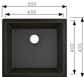
S510-U450 Onderbouwspoeltafel 450 Onderkast: 600 mm # 43431, -170, -290, -380 # 43927000 Manuele lediging # 43937000 Automatische lediging
