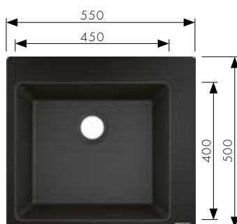
S510-F450 Inbouwspoeltafel 450 Onderkast: 600 mm # 43312, -170, -290, -380 # 43927000 Manuele lediging # 43937000 Automatische lediging
