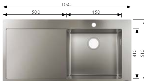
S715-F450 Inbouw en vlakkbouw spoelbak met afdruiplak diepte 190 mm, voor inbouwkast: 600 mm # 43306, -800, met een kraangat # 43920000 Manuele lediging
