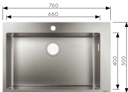
S711-F660 Inbouw en vlakkbouw spoeltafel diepte 190 mm, voor inbouwkast: 800 mm # 43302, -800, met een kraangat # 43921000 Manuele lediging
