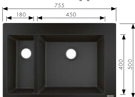
S510-F635 Inbouwspoeltafel 180/450 Onderkast: 800 mm # 43315, -170, -290, -380 # 43928000 Manuele lediging # 43938000 Automatische lediging
