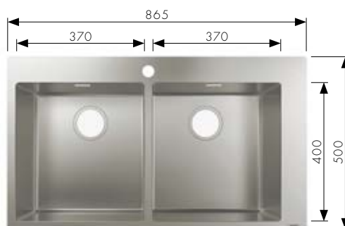
S711-F765 Inbouw en vlakkbouw spoeltafel diepte 190 mm, voor inbouwkast: 900 mm # 43303, -800, met kraangat # 43922000 Manuele lediging
