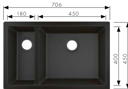
S510-U635 Onderbouwspoeltafel 180/450 Onderkast: 800 mm # 43433, -170, -290, -380 # 43928000 Manuele lediging # 43938000 Automatische lediging
