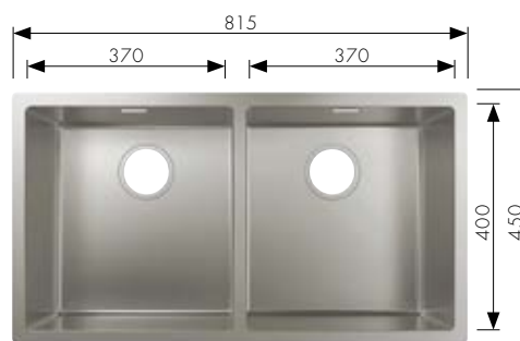
S719-U765 Onderbouw spoeltafel diepte 190 mm, voor inbouwkast: 900 mm # 43430, -800 # 43922000 Manuele lediging # 43932000 Automatische lediging
