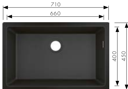
S510-U660 Onderbouwspoeltafel 450 Onderkast: 800 mm # 43432, -170, -290, -380 # 43927000 Manuele lediging # 43937000 Automatische lediging
