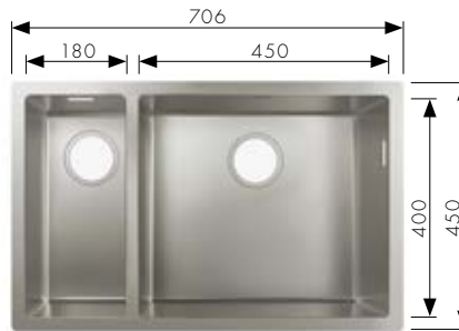
S719-U655 Onderbouw spoeltafel diepte 190 mm, voor inbouwkast: 800 mm # 43429, -800 # 43924000 Manuele lediging # 43934000 Automatische lediging
