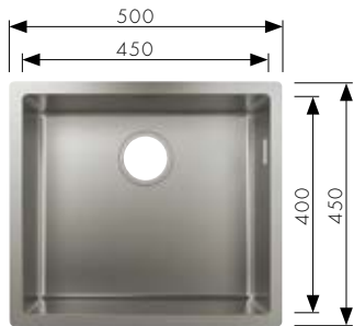
S719-U450 Onderbouw spoeltafel diepte 190 mm, voor inbouwkast: 600 mm # 43426, -800 # 43920000 Manuele lediging # 43930000 Automatische lediging
