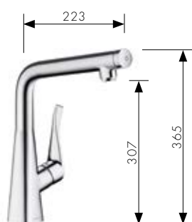
M712-H320 Select ééngreeps keukenmengkraan 320 met draaibare uitloop # 73810, -000, -800
