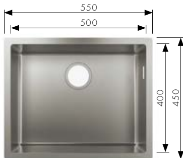
S719-U500 Onderbouw spoeltafel diepte 190 mm, voor inbouwkast: 600 mm # 43427, -800 # 43926000 Manuele lediging # 43936000 Automatische lediging
