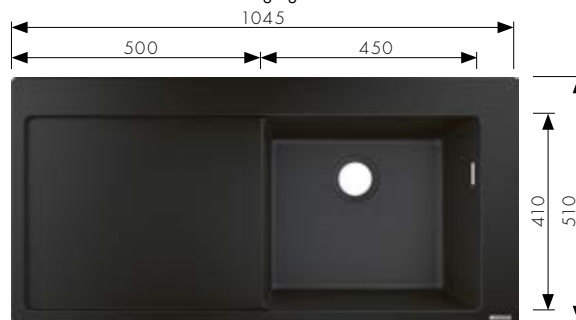
S514-F450 Inbouwspoeltafel 450 met afdruiplak Onderkast: 600 mm # 43314, -170, -290, -380 # 43927000 Manuele lediging # 43937000 Automatische lediging
