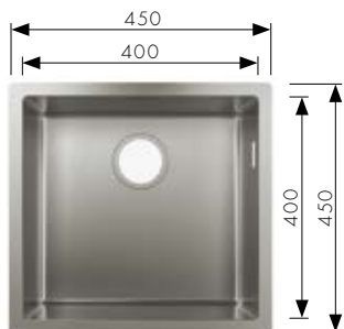
S719-U400 Onderbouw spoeltafel diepte 190 mm, voor inbouwkast: 500 mm # 43425, -800 # 43920000 Manuele lediging # 43935000 Automatische lediging
