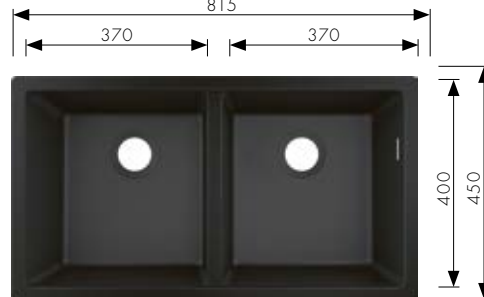
S510-U770 Onderbouwspoeltafel 370/370 Onderkast: 900 mm # 43434, -170, -290, -380 # 43928000 Manuele lediging # 43938000 Automatische lediging
