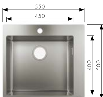
S711-F450 Inbouw en vlakkbouw spoeltafel diepte 190 mm, voor inbouwkast: 600 mm # 43301, -800, met een kraangat # 43920000 Manuele lediging
