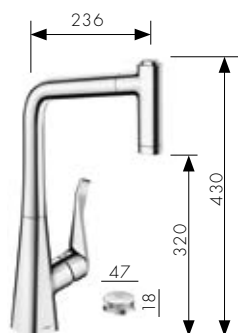
M7120-H320 2-gats ééngreeps keukenmengkraan 320 met uittrekbare vuistdouche en aparte Select-knop, 2 straalsoorten # 73806, -000, -800
