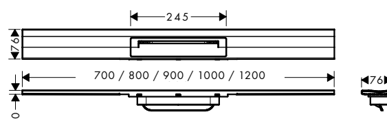
RainDrain Flex voor montage tegen de wand
