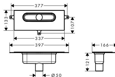
uBox universal voor verticale installatie
