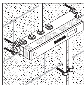
Installation murale ; ici avec entretoises variables et vis à double filetage M10
