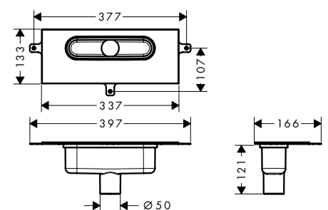
uBox universal für vertikale Installation
