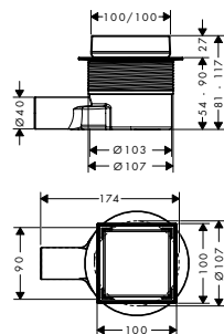
RainDrain Point Rost rückseitig befliesbar 100 x 100
