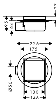
RainDrain Spot Rost rückseitig befliest
