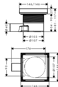
RainDrain Point Rost rückseitig befliesbar 150 x 150
