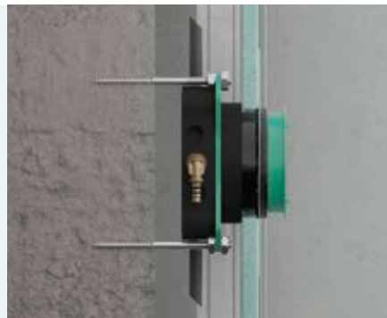
Installation vor der Wand
