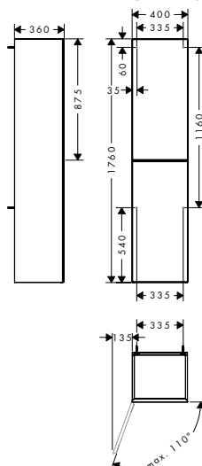
Charnière de porte gauche
