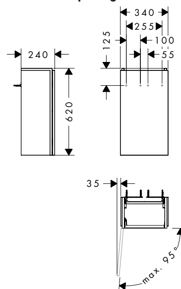
Charnière de porte gauche
