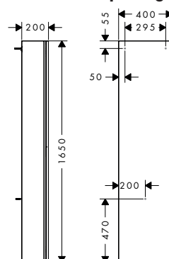
Charnière de porte gauche
