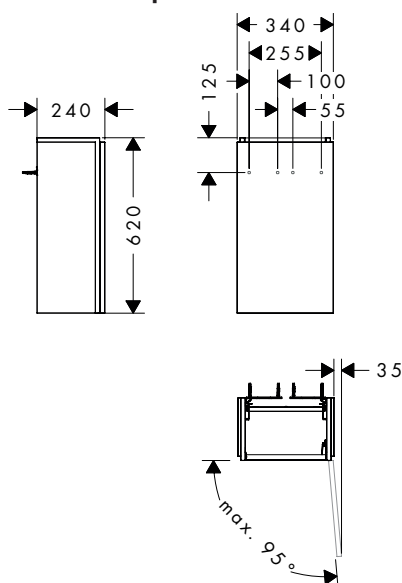
Charnière de porte droite
