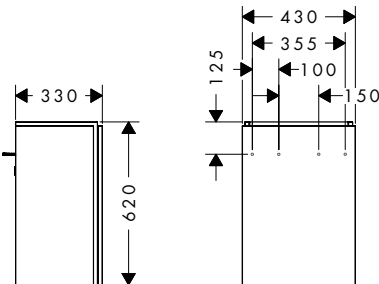
Charnière de porte gauche
