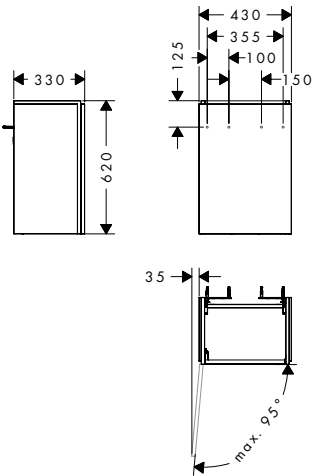
charnière de porte gauche
