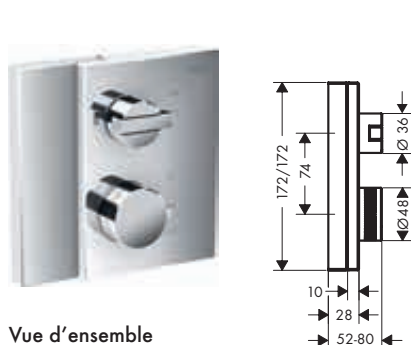
coupe diamant
