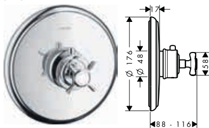
poignée croisillon
