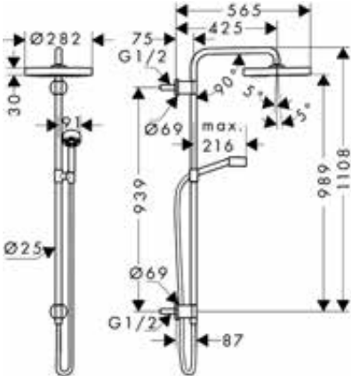
Colonne de douche 280 1jet pour installation encastrée
