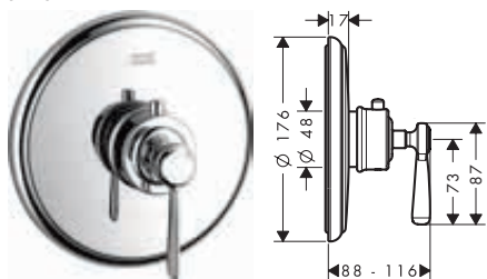
poignée manette
