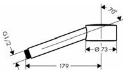
Douchette à main 75 ljet
