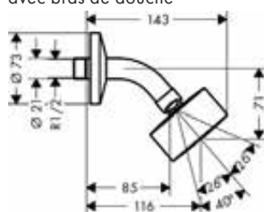
Douche de tête 280 2jet avec bras de douche
