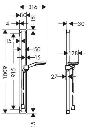
Set de douche 0,90 m avec douchette à main 120 3jet
