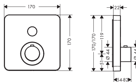
Thermostat softsquare encastré pour 1 fonction
