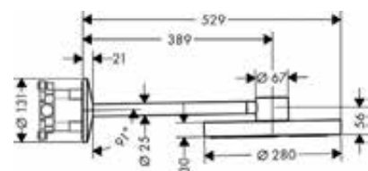
Douche de tête 75 ljet EcoSmart avec bras de douche
