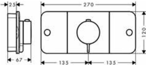
Module thermostatique encastré avec 2 sorties
