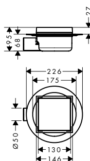
RainDrain Spot vendbart kvadratisk afløb
