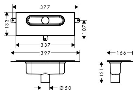
uBox universal til lodret installation
