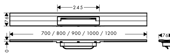
RainDrain Flex mod bagvæg
