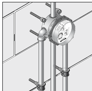
Montering foran væggen – her med variable afstandsstykker på hængebolte M 10
