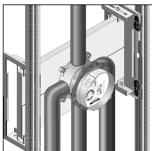
Montering på bæresystem
