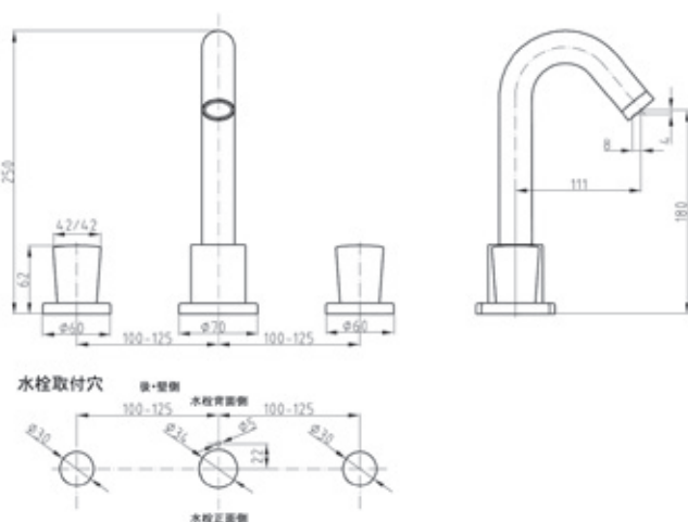
71300000 ロギス 3ホールリム付式バス混合水栓(化粧部)
