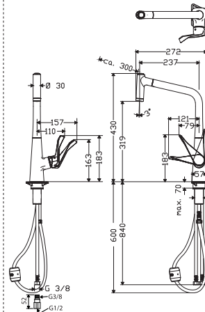
34822000 アクサーチッテリオ M 2ホール引出式 キッチンシャワー混合水栓 220
