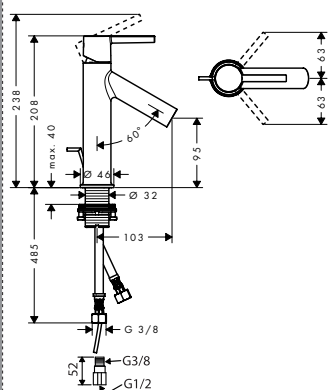
10117000 アクサースタルク シングルレバー 洗面混合水栓 90 (ポップアップ引棒無)
