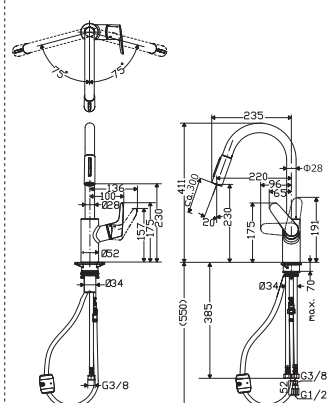
39862004 アクサーチッテリオセレクト シングルレバー 引出式キッチンシャワー混合水栓 230
