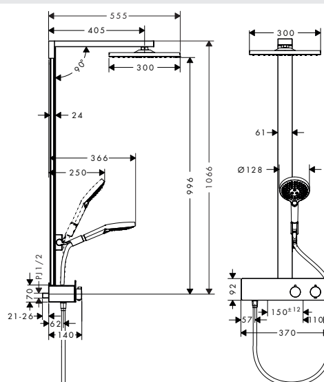
27361000 レインダンスE シャワーパイプ 300 1ジェット ST300
