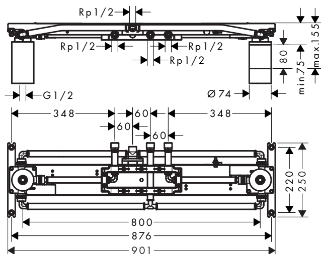
10922180 埋込部 シャワーヘッド 1200 / 300用
