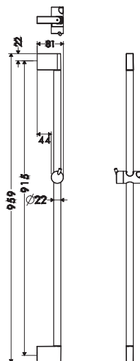
27980000 アクサースタルク シャワーセット 900
