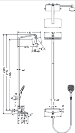
27113400 レインダンスE シャワーパイプ 360 1ジェット スバウト付
