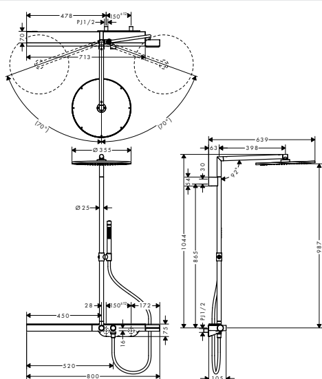
27984000 アクサーシャワー シャワーパイプ 800サーモスタット / 350オーバーヘッドシャワー
