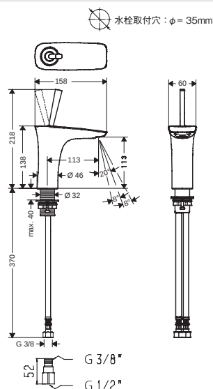
15074000 ブラビダ シングルレバー洗面混合水栓 110 (ポップアップ引棒有)
