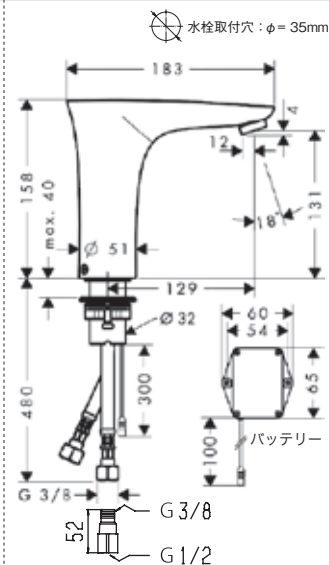
15170400 ブラビダ 自動洗面混合水栓 温度調節付 ホワイト・クロム
