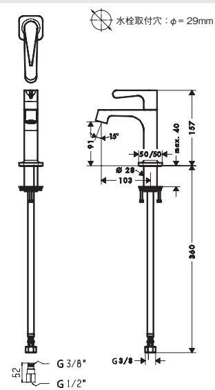
34130000 アクサーチッテリオM 単水栓 90
