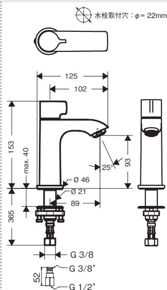
45130000 アクサーウノセレクト 単水栓 80
