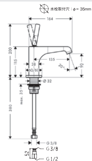
71120000 ロギス 単水栓 70 (ポップアップ引棒無)
