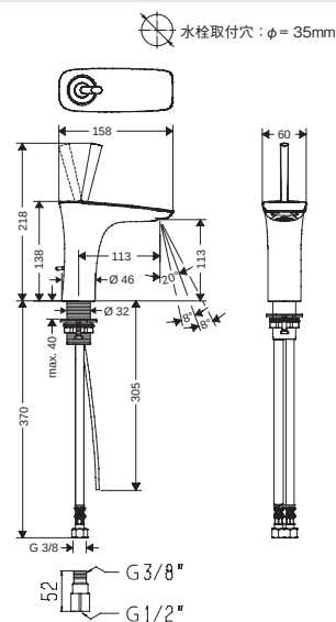
15170400 ブラビダ 自動洗面混合水栓 温度調節付 ホワイト・クロム
