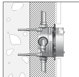
Installatie voor de wand, gebruik makend van afstand draadeinden.
