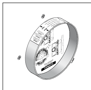
Installatie prefab wandpanelen
