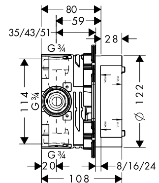
iBox® universal vooraanzicht en zij aanzicht
