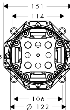
iBox® universal vooraanzicht en zij aanzicht
