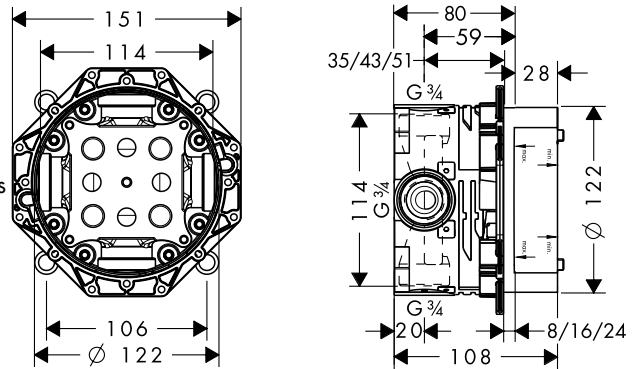
iBox® universal vooraanzicht en zijaanzicht
