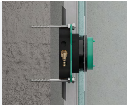
Instalación fuera de la pared
