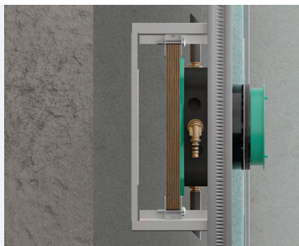
Instalación sobre un sistema de soporte
