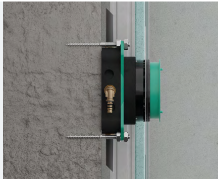
Instalación sobre la pared
