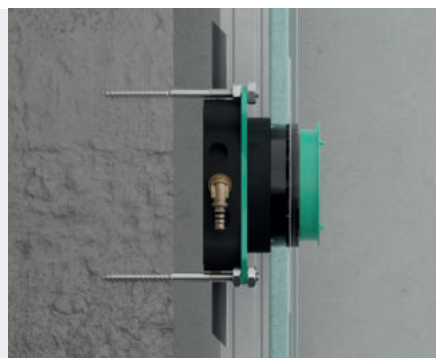
Installation devant le mur
